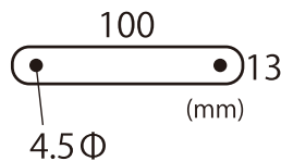
補強用小型バー
