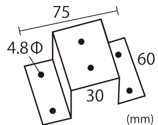
30×30角材取付用
